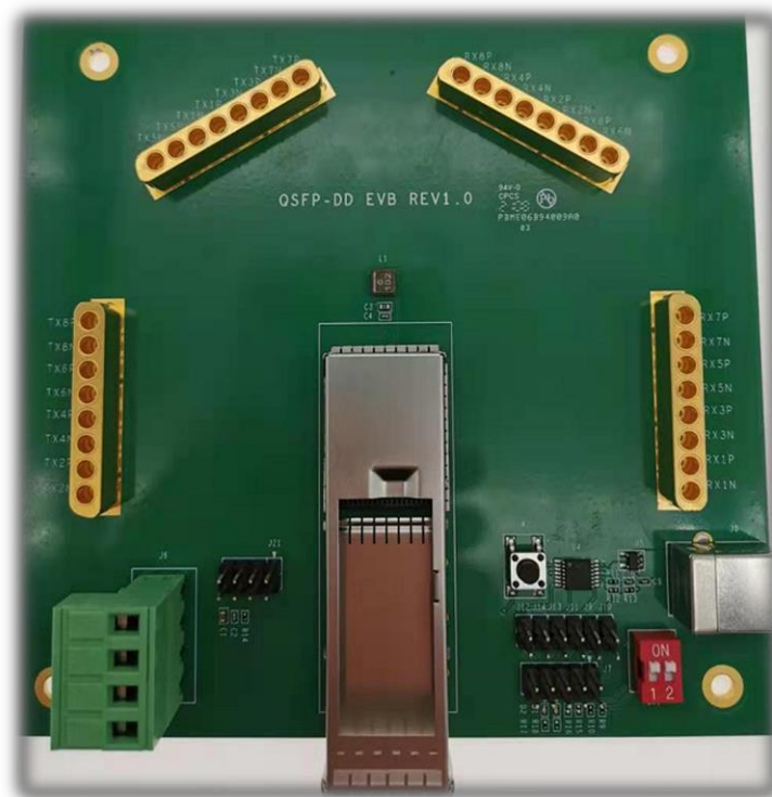
Figure1: QSFPDD-MCB-8
