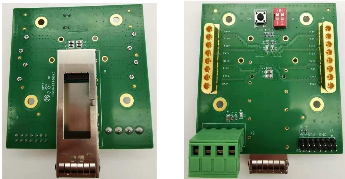
Figure1: QSFP28-MCB-8-IL
