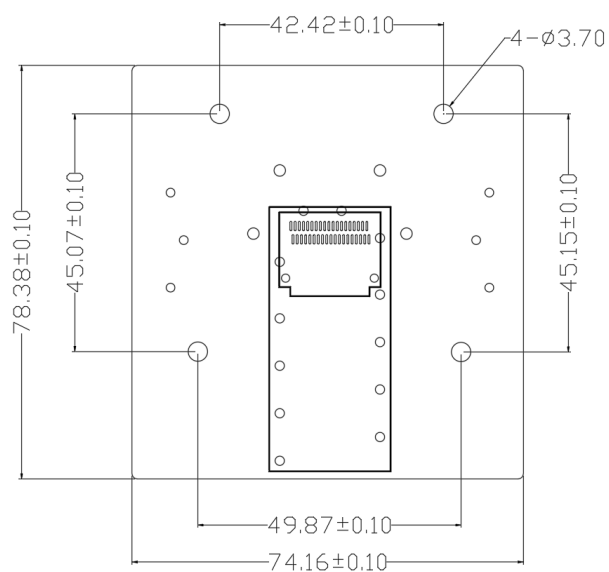
Figure1: QSFP28-MCB-8-IL
